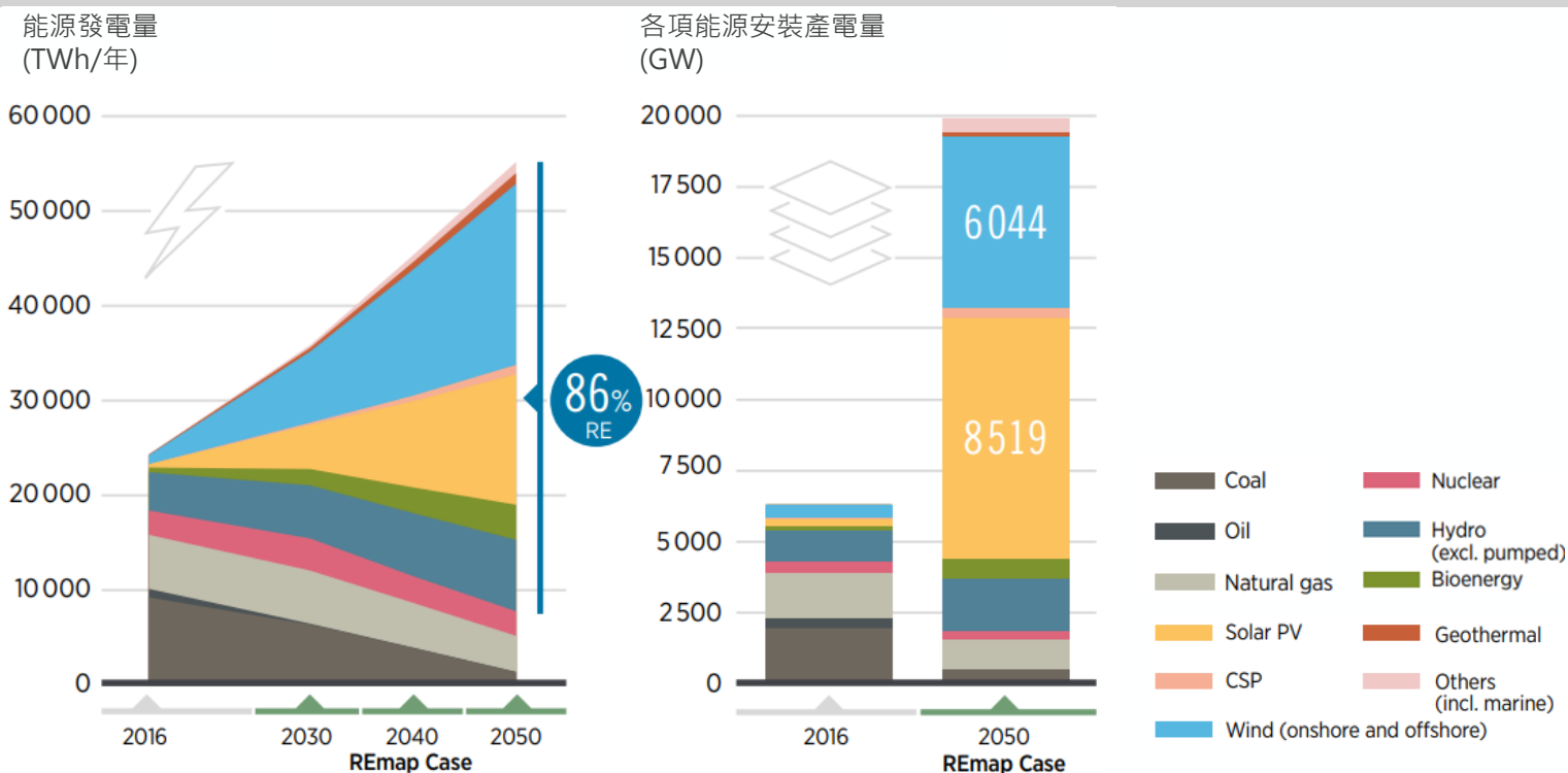
各項能源發電量和總裝機量產生之能源總量
