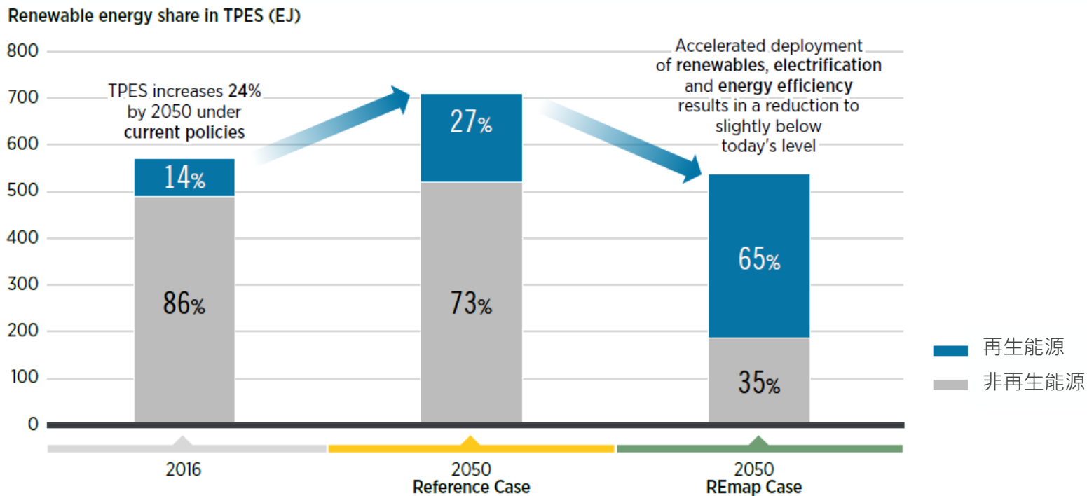
再生與非再生能源占主要能源供應源比率 (2016-2050)
