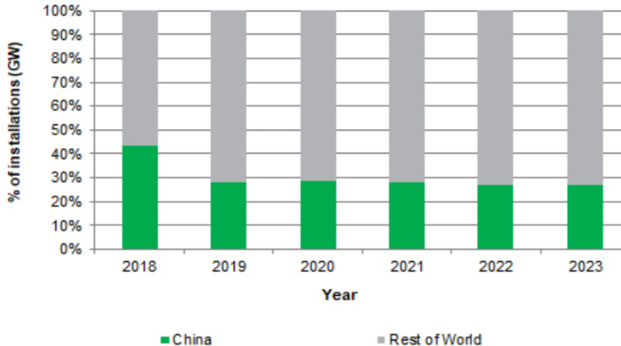
全球太陽能安裝量(中國 vs. 其他區域)
