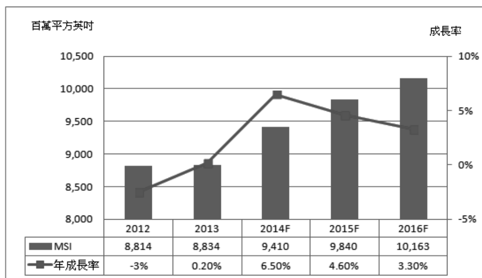
圖九 2014 年~2016 年矽晶圓出貨量
